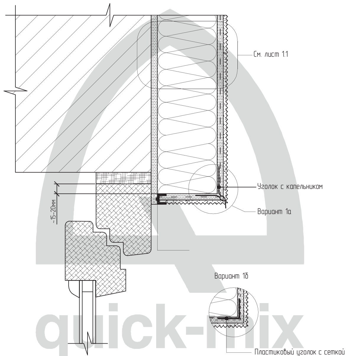
Вертикальный разрез
